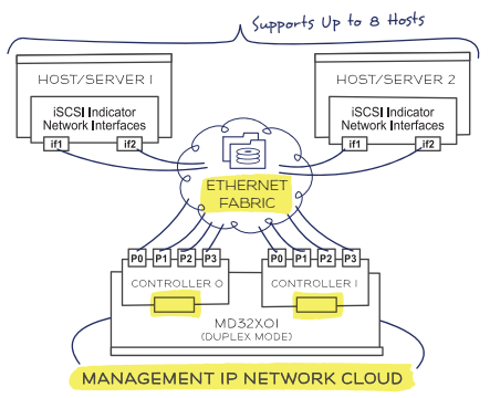
ISCSI CONFIGURATION
